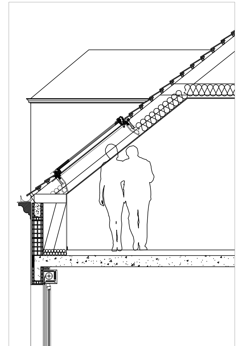
Volume sous brisis en coupe
