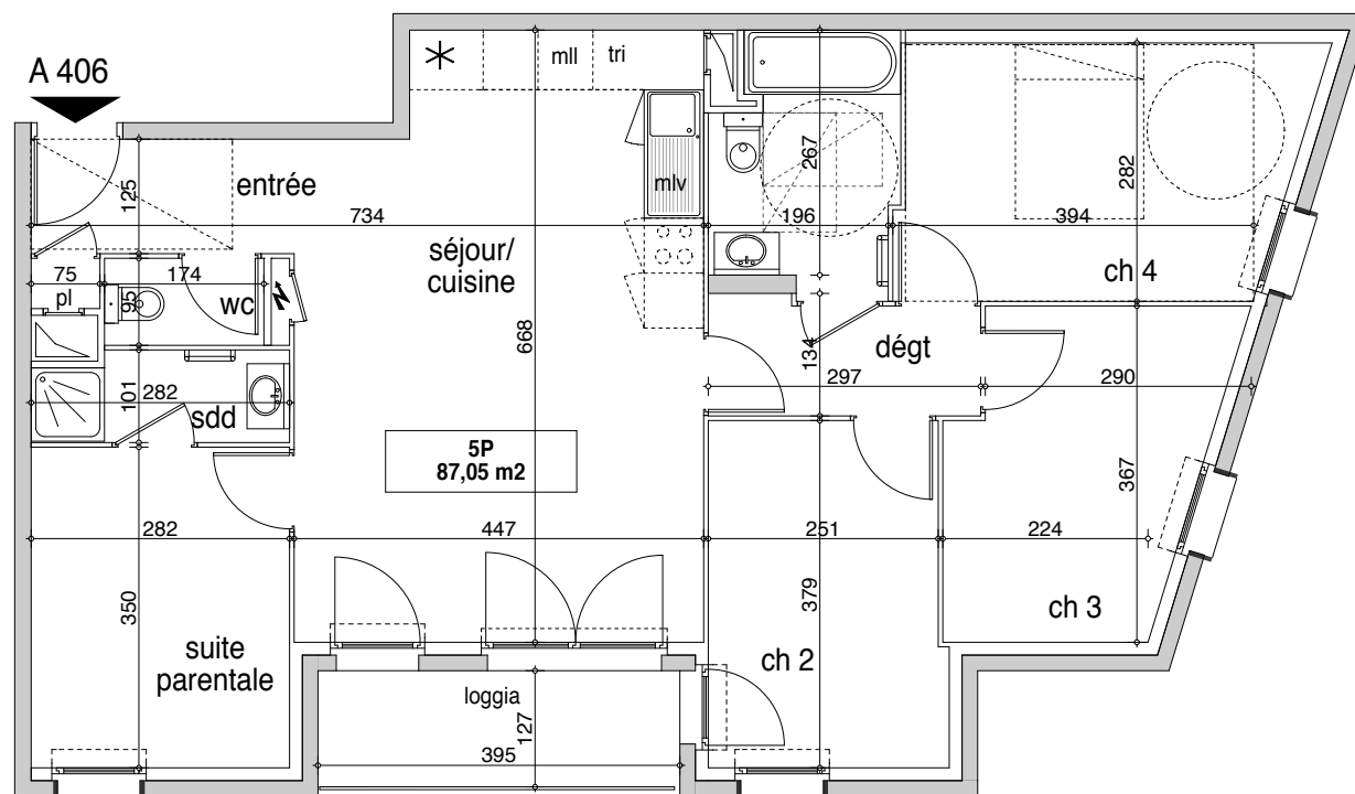
plan provisoire
