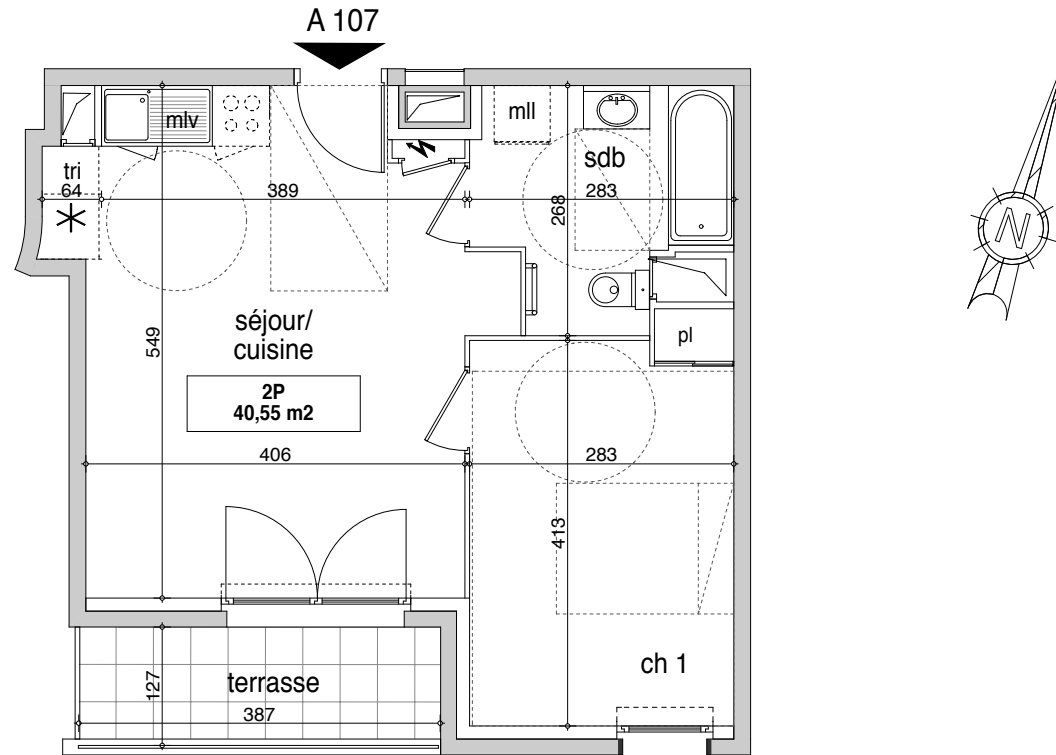
plan provisoire
